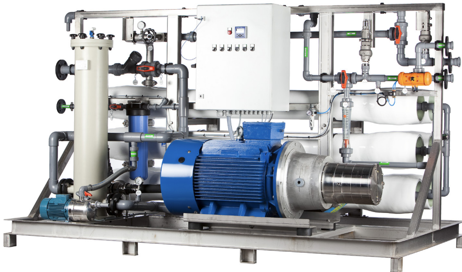
Ett exempel av Enwa's SRH serie - 200 m 3 /24tim
